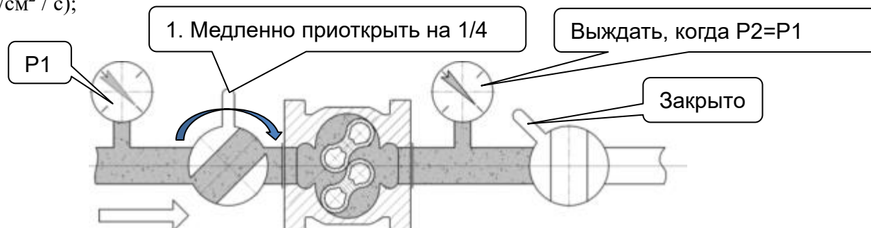
Рисунок 11. Начальное открытие запорного устройства.
