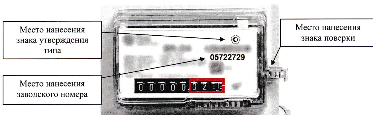
Рисунок 2 – Схема пломбировки от несанкционированного доступа, обозначение места нанесения знака поверки, место нанесения заводского номера и знака утверждения типа
