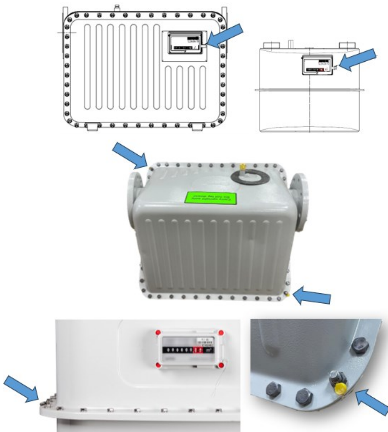
Рисунок 3 – Схема пломбировки
